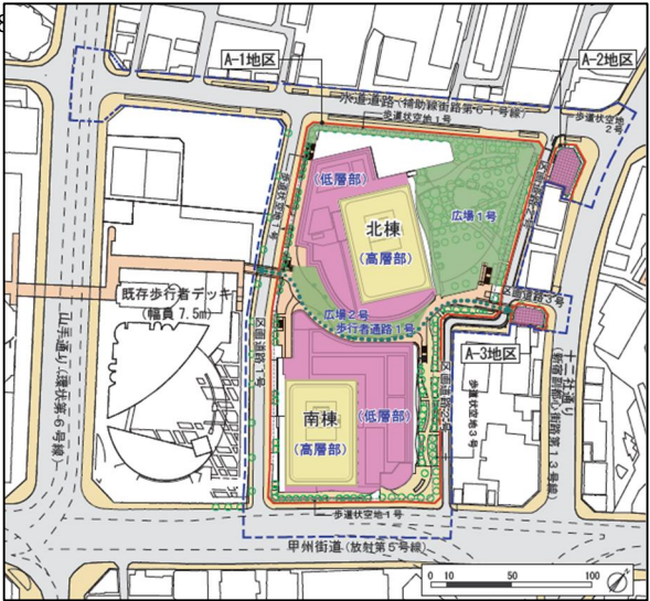
【開発事業予定区域 敷地配置図】
