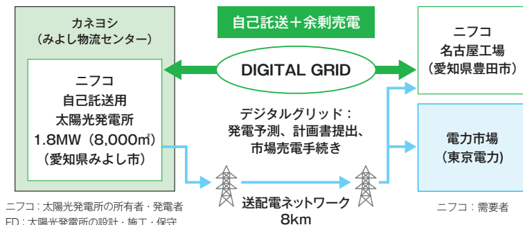
カネヨシみよし物流センター屋上に設置された太陽光発電所
