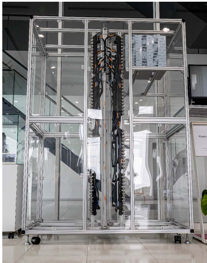
（写真左上：データセンター向け水冷冷却装置、左中：水冷サーバー用クーリングプレート、左下：バルブ機能付き継手、右：スーパーコンピュータ「富岳」向け水冷冷却用樹脂配管製品）
