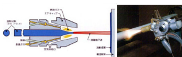
溶棒式フレイム溶射（燃焼ガス）
