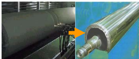
溶射中 仕上げ後 製紙ロールへのWCサーメット溶射
