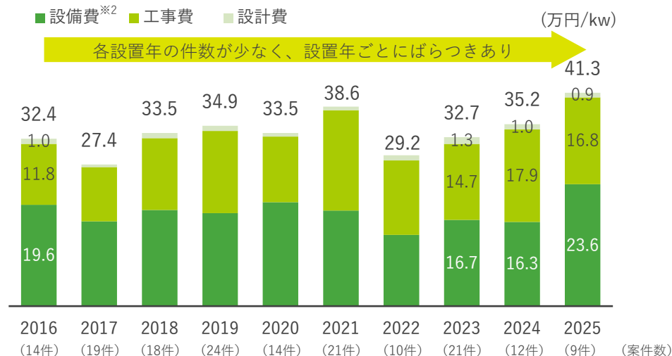
陸上風力発電 資本費推移 (設置年度別)
