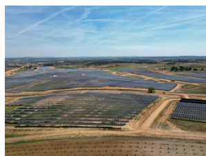
バルデカレタス太陽光発電所 (スペイン) 定格容量: 38MW (2023年12月商業運転開始)
