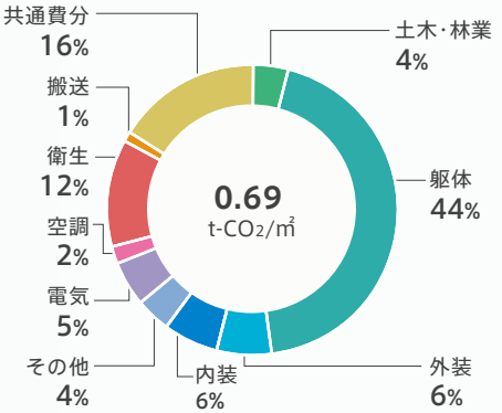
ブランズタワー大阪本町における 排出量試算によるCO 2 割合
