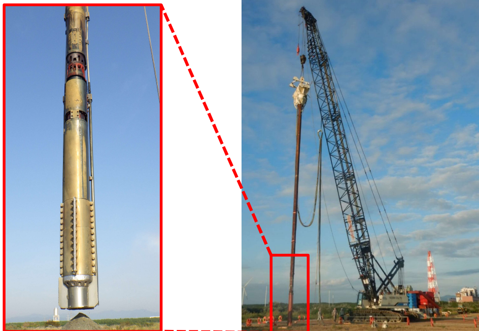
高周波振動機(バイブロフロッタ)
