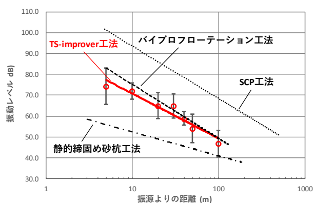
図3 振動の距離減衰
