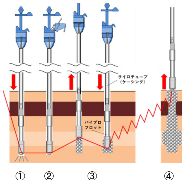
図1 改良杭造成手順
