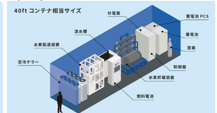
「Hydro Q-BiC Lite」基本構成
