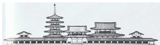
法隆寺西寺院立面図 出典:彰国社「日本の都市空間」
